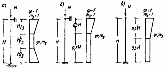
Рис. 4. Коэффициенты \varphi и m_g по высоте сжатых стен и столбов
