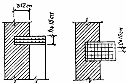
Рис. 13. Железобетонные распределительные плиты
