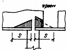
Рис. 16. Эпюра распределения давления в кладке висячих стен при наличии проема
