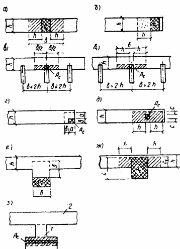
Рис. 9. Определение расчетных площадей сечений при местном сжатии
