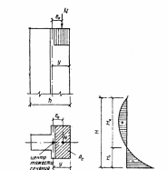
Рис. 5. Внецентренно сжатие
