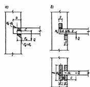
Рис. 14. Расчетные схемы заделки консольных балок.
