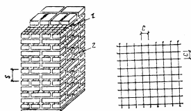
Рис. 10. Поперечное (сетчатое) армирование каменных конструкций
